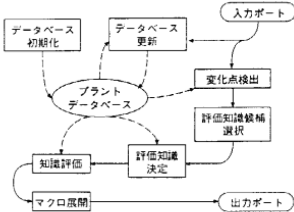
図4: アクション部の内部構造
