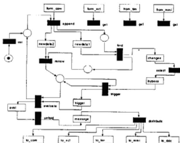
図 6: アクション部のベトリネット表現
