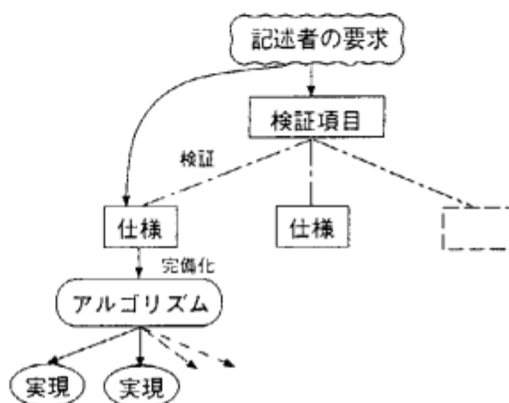
図 5: 仕様と検証項目の関係
