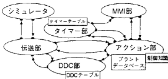
図 3: オブジェクト構成
