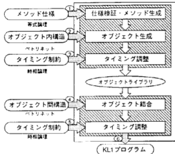
図 1: プログラム生成の流れ
