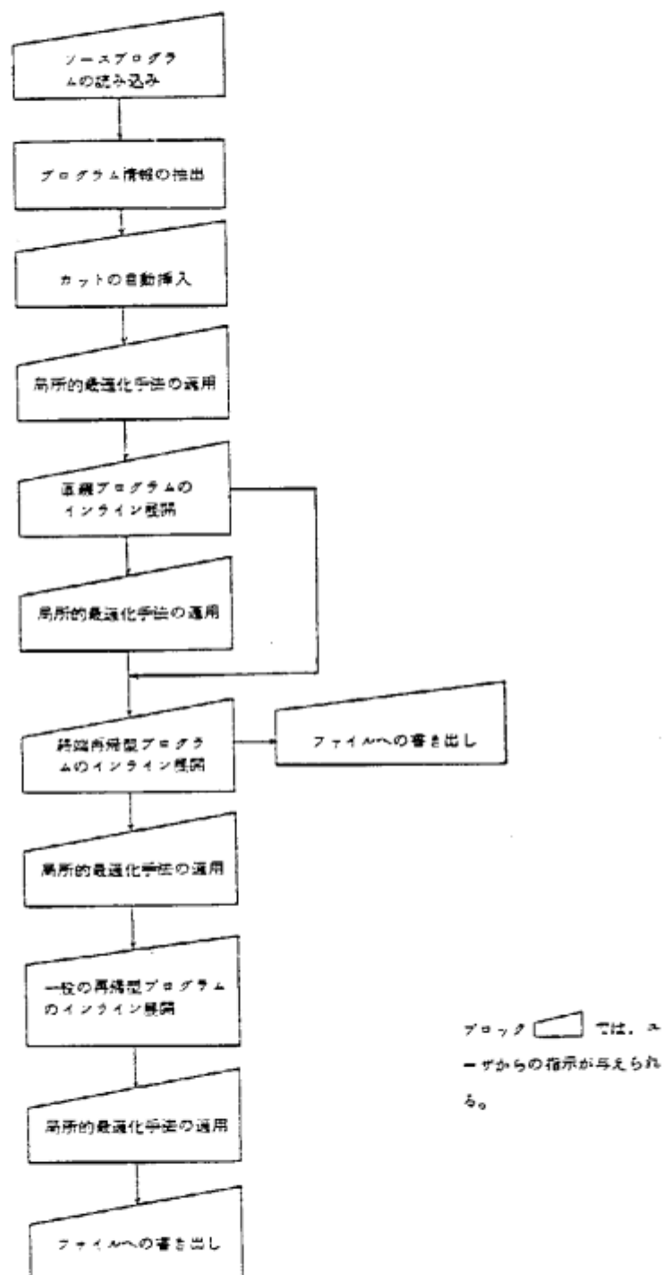
図1 Prologソースレベル・オブティマイザの手続きの流れ Fig. 1 Procedural flow of the Prolog optimizer
