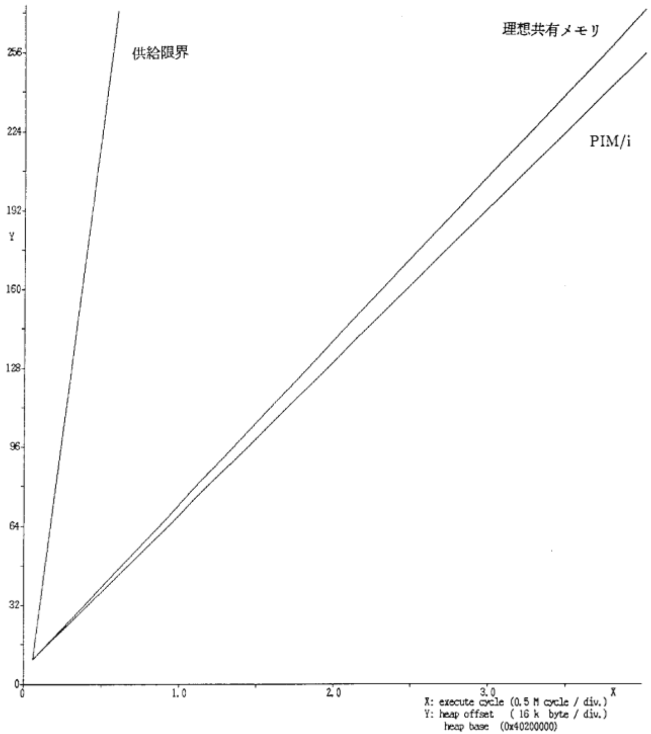
図 2: 時間とメモリ使用量の関係
