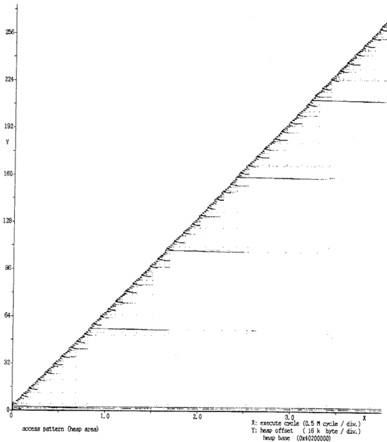
図 1: メモリ割り当ての様子
