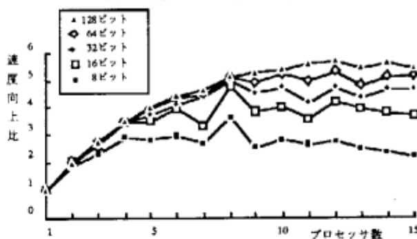
図4 速度向上比 (比較器)
