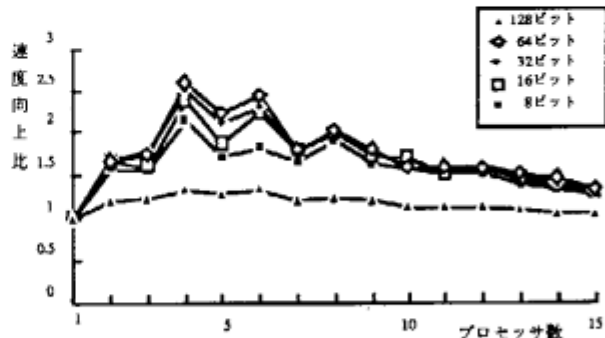
図5 速度向上比 (マルチプレクサ)
