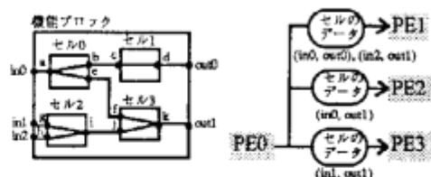
図1 機能ブロックの構成図 図2 割り付けの例
