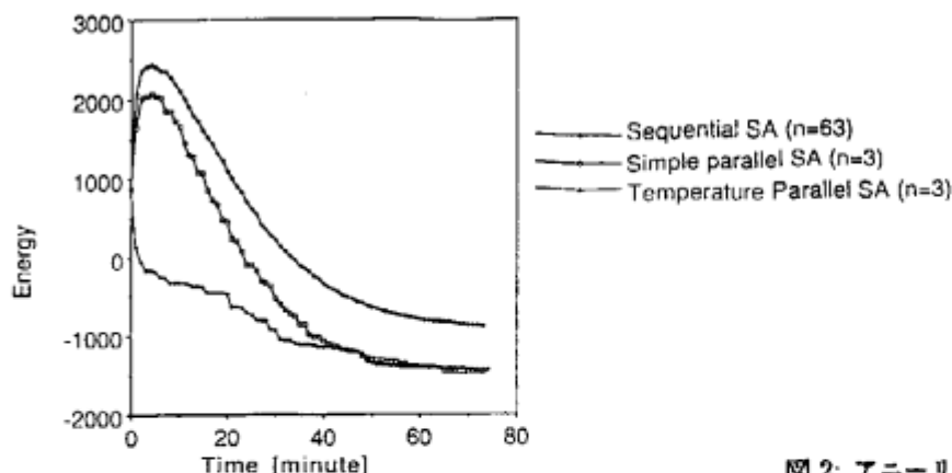
図 2: アニーリング経過の比較
