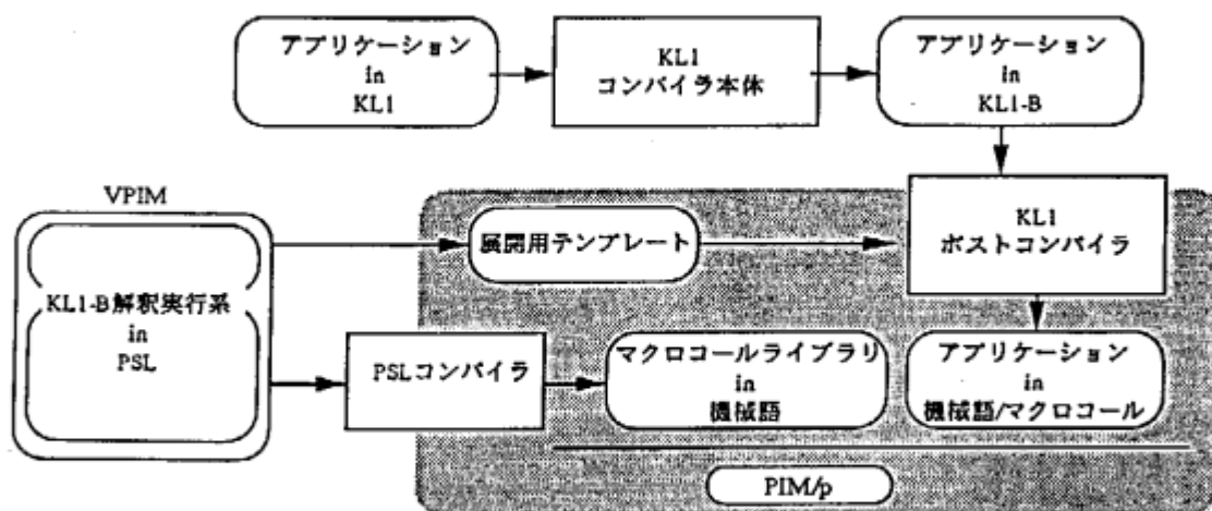
図 2 KL1プログラム実行
