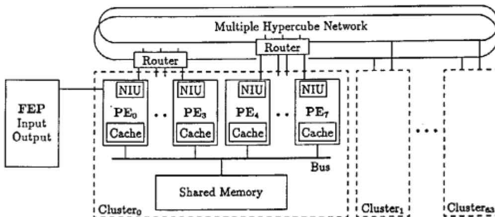
図1: PIM/pの全体構成
