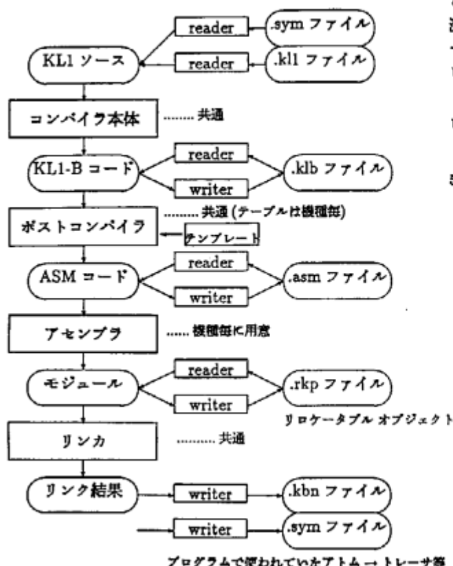
図 5: KL1 コンパイラの全体構成
