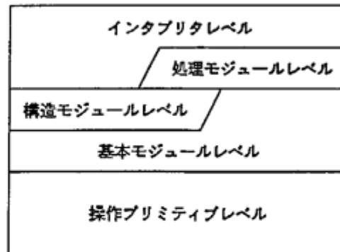
図 3: VPIM の階層
