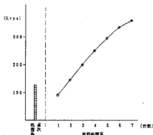
図7 n-reverse (1000要素)・測定結果
