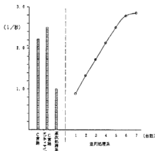
図6 2進木データベース・測定結果
