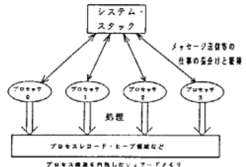
図4 並列処理
