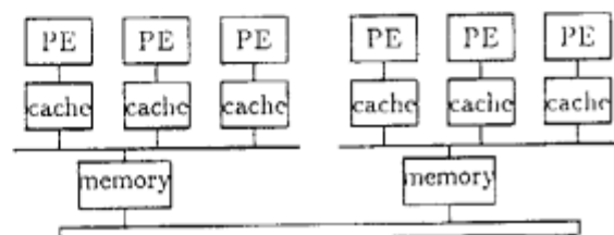
図 2: クラスタ間共有メモリ方式 (2)
