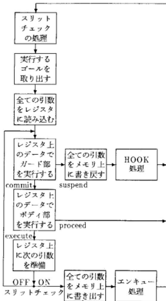
図 1: 従来の KL1-B のゴール実行方式
