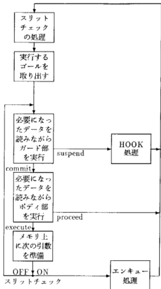
図 2: 新しい KL1-B のゴール実行方式
