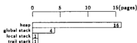
図 7: エリア別使用ページ数
