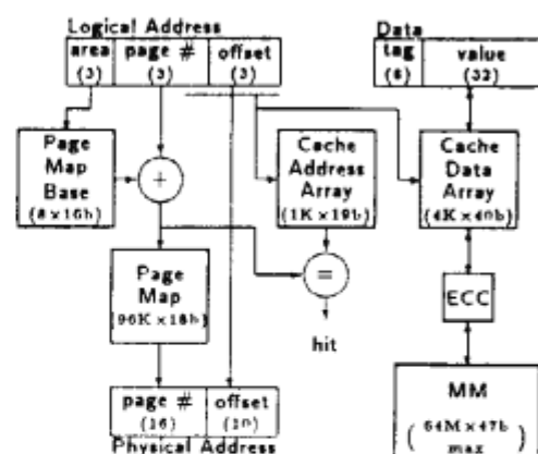
図 1: PSI-II のメモリ・システム
