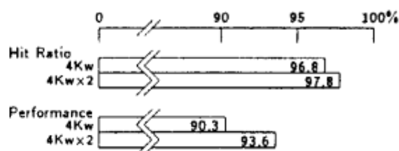
図 4: 容量削減の影響
