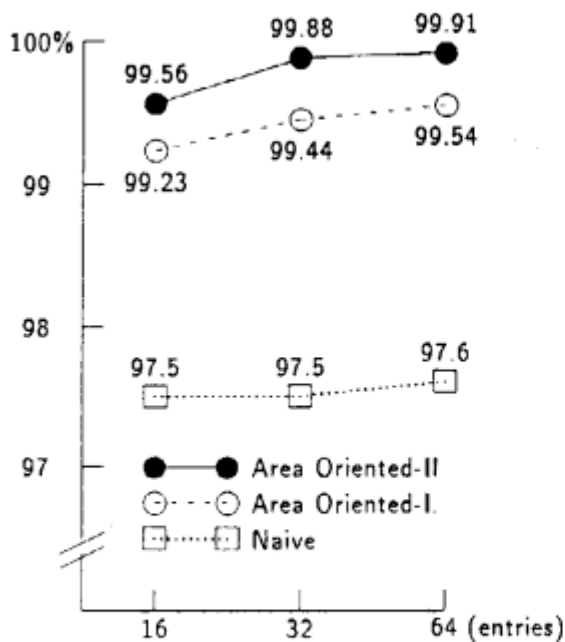
図 8: データ用アドレス変換バッファのヒット率
