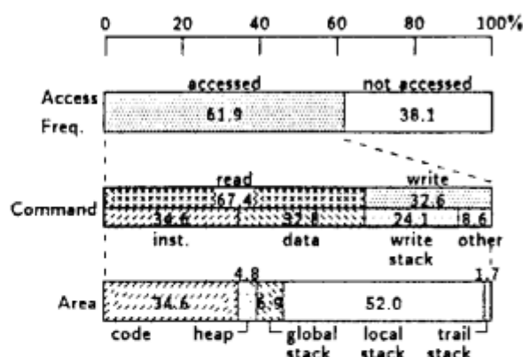
図 2: アクセス頻度
