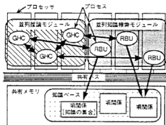
図1 試作システムの構成
