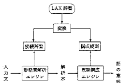
図1: 形態素意味解析の流れ
