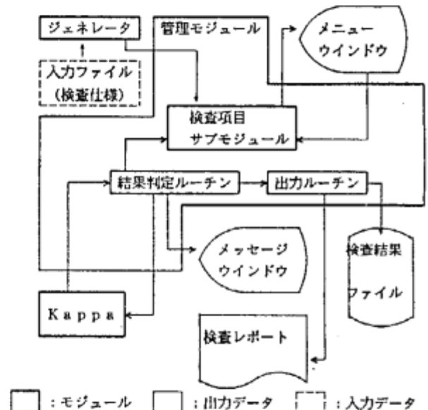
図1 検査システムの構成
