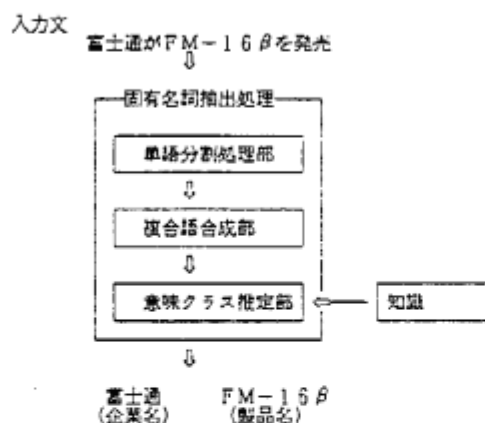
図1 固有名詞抽出処理の概要
