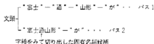
図2 未登録固有名詞を含んだ入力文字列の解析例
