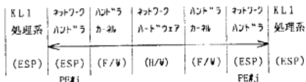
図5. ネットワークの階層構造
