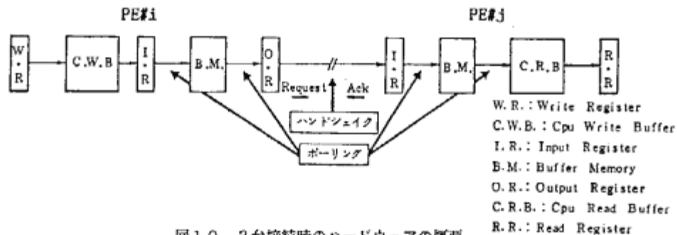
図10. 2台接続時のハードウェアの概要
