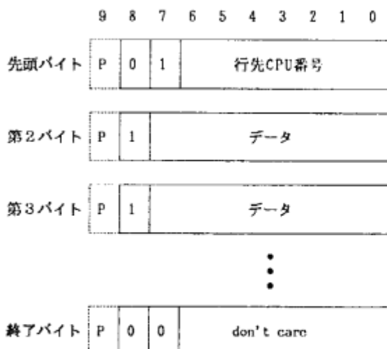
図4. パケット形式
