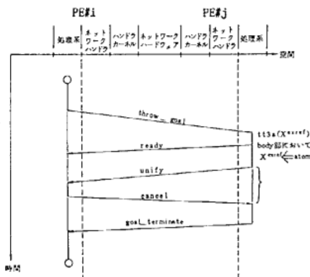
図7. メッセージ（通信オーダ）交換の概念図
