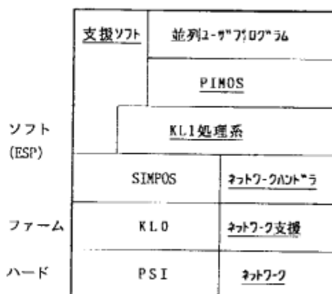
図2. マルチPSI第1版のシステム階層構成
