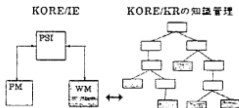
図3. KORE/IE と KORE/KR の協調
