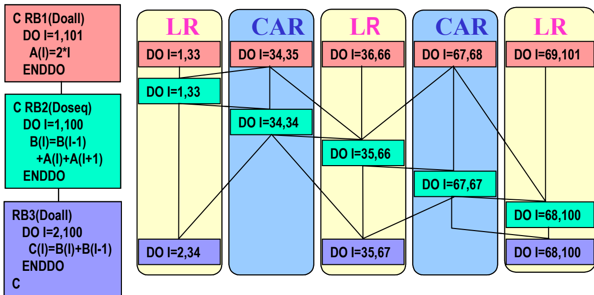
図 7 データローカライゼーションにおける整合分割
