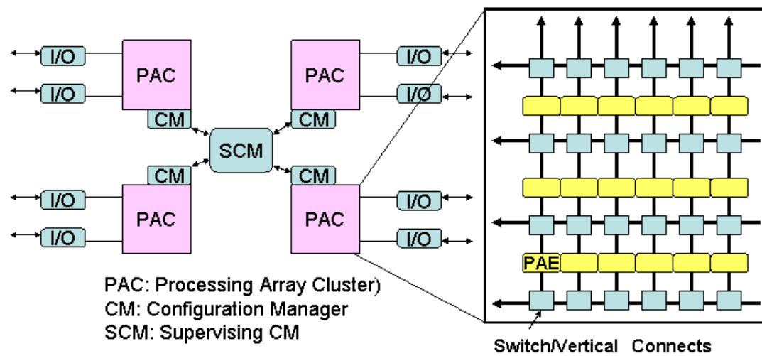
図 2 PACT XPP の構成
