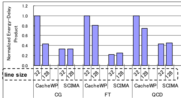
図 11 ED 積 (fig9, SWoPP02)
