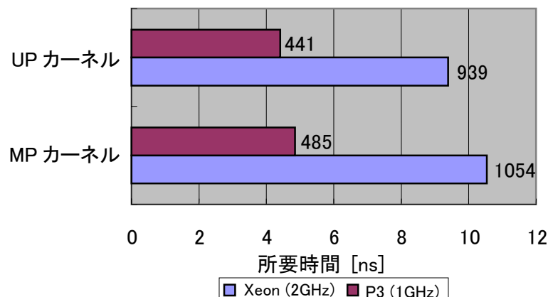
図4 gettimeofday()処理の実行時間
