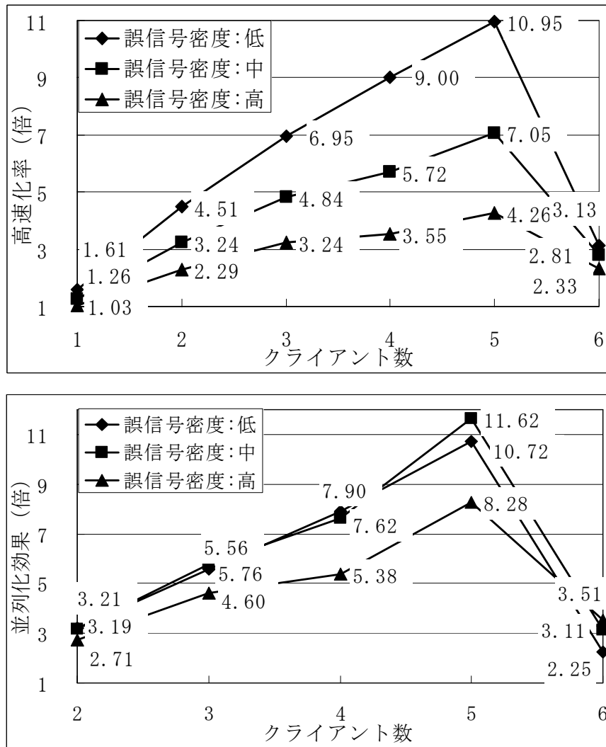
図 10 全実行時間の高速化率と仮説生成部分の並列化効果
