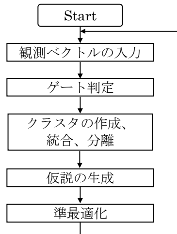
図 3 航跡型 MHT の処理フロー
