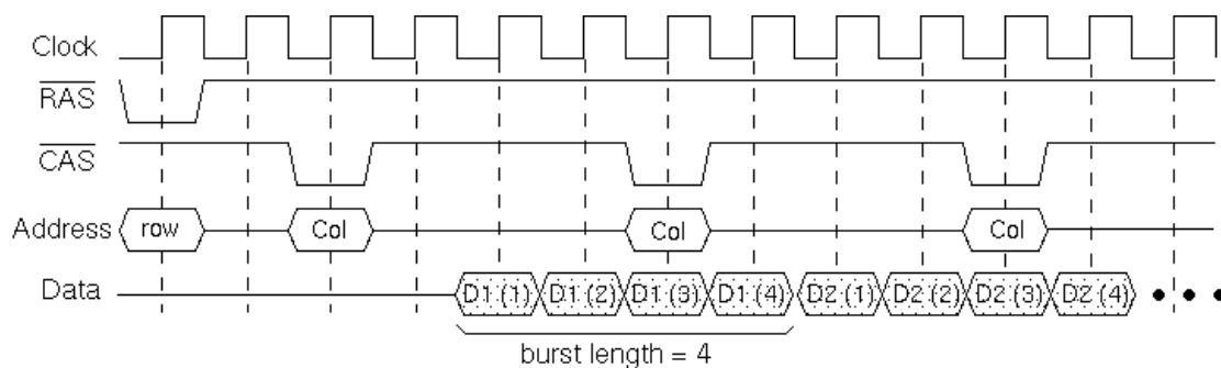
図 5 SDRAM のアクセスタイミング
