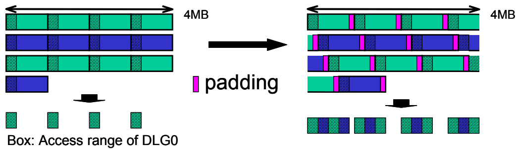
図 9 配列間パディングを用いたラインコンフリクトの除去
