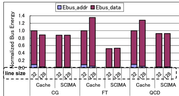
図 7 バスの消費エネルギー
