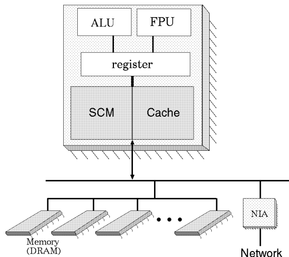
図 1 SCIMA の構成図
