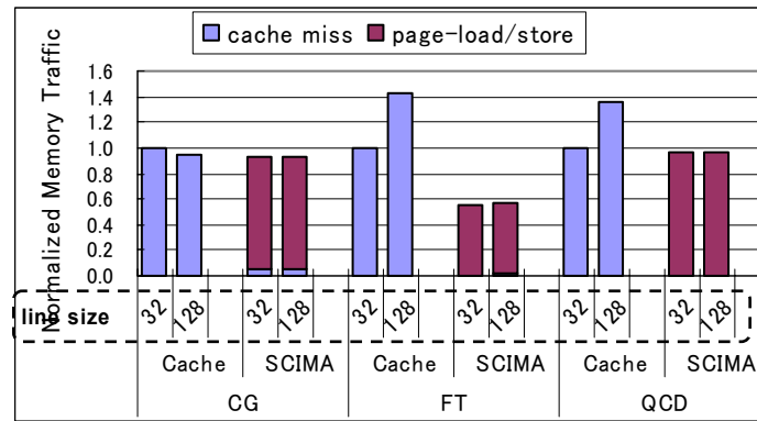
図 6 メモリトラフィック
