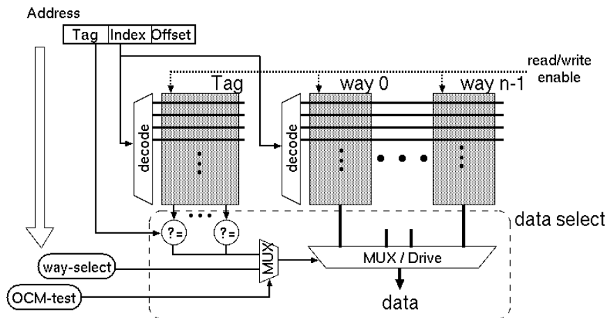
図 3 SCIMA の SCM アクセス
