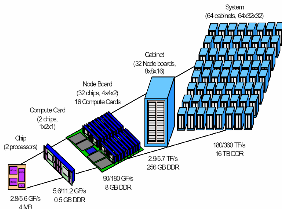
図 2.3 Blue Gene/L の構成概念図 (出典: 文献[1])
