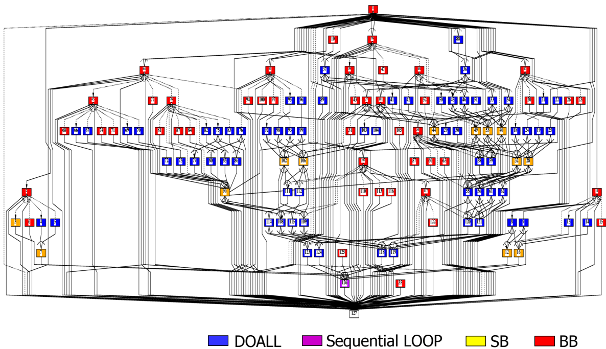
図 6 図 5 の LOOPS 部分のマクロタスクタスクグラフ
