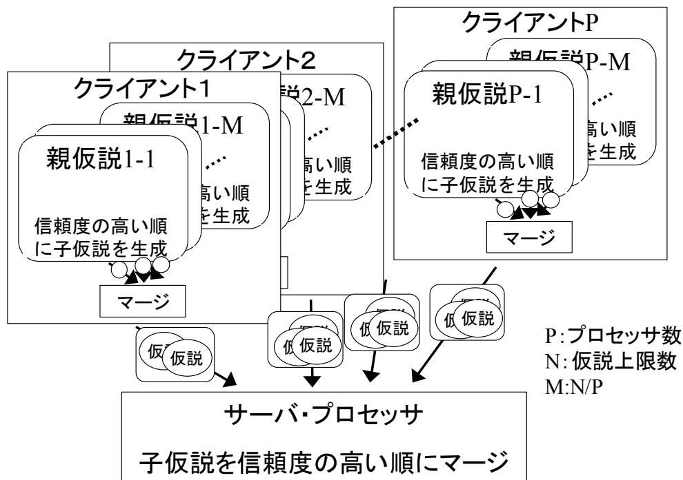
図 8 仮説生成の並列化
