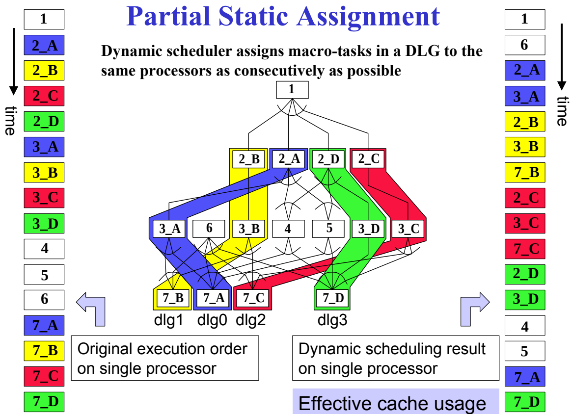
図 8 データローカライゼーショングループ DLG と 1 プロセッサへのスケジューリング例
