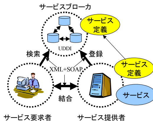
図1 Web サービスアーキテクチャ
