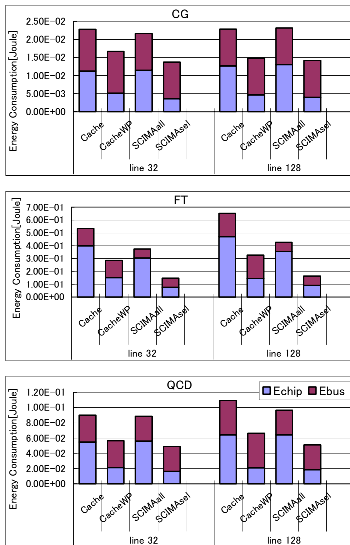
図 9 メモリシステム全体の消費エネルギー
