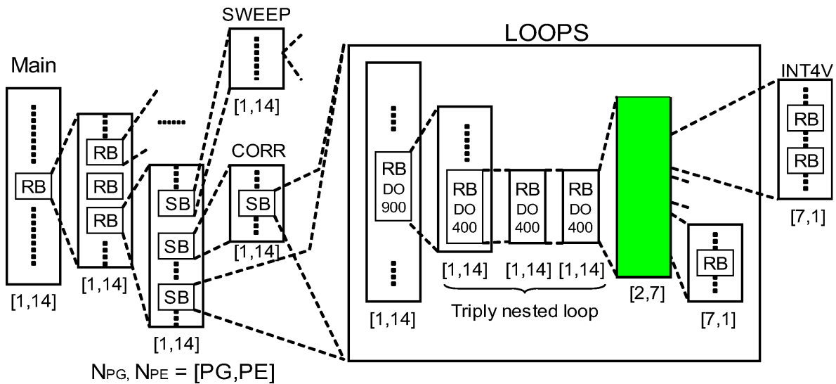
図5 SPEC CFP95 SU2COR における並列処理階層及びプロセッサグループ(PG)数、PG内プロセッサ数の自動決定
