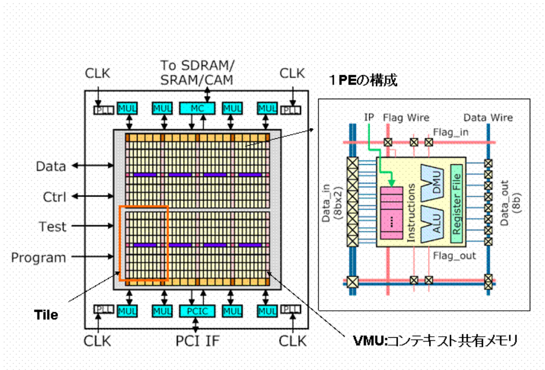
図1 DRP-1の構成
