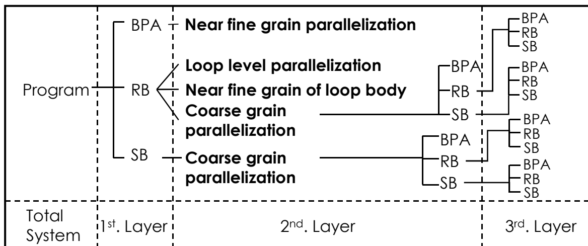
図2 マクロタスクの階層的定義
