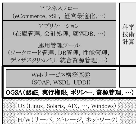
図 4 OGSA の位置づけ
