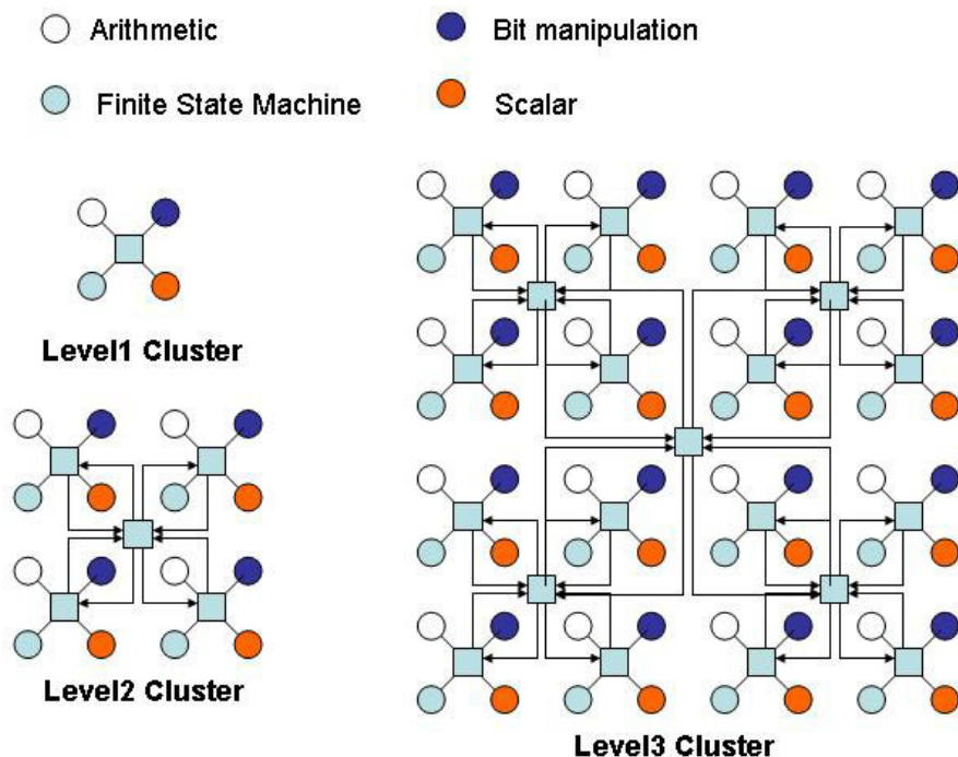
図 3 Quicksilver ACM の構造
