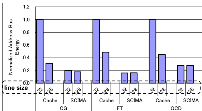
図 8 アドレスバスの消費エネルギー
