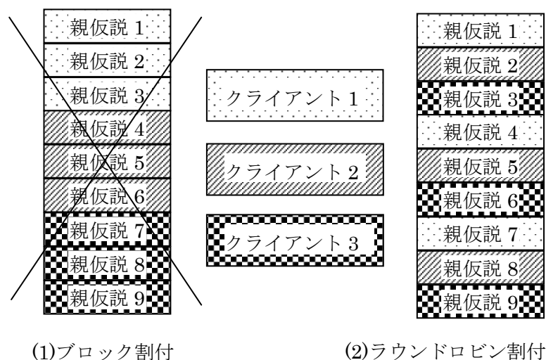
図 9 親仮説の分配方法
