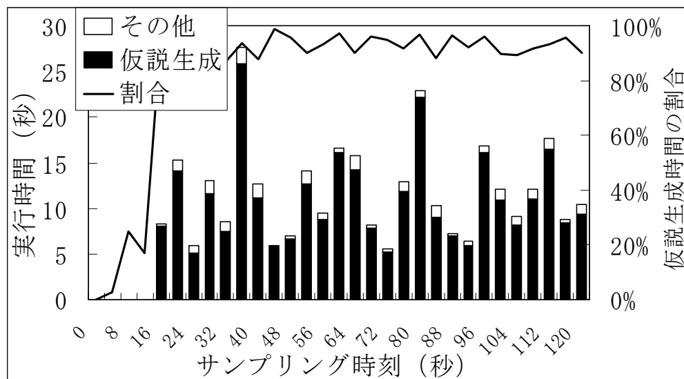
図 7 各サンプリング時刻毎の実行時間
