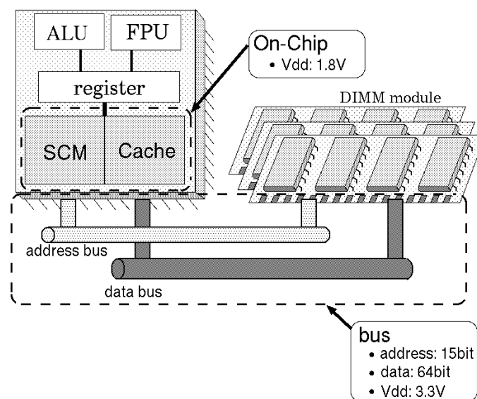
図 4 評価モデル
