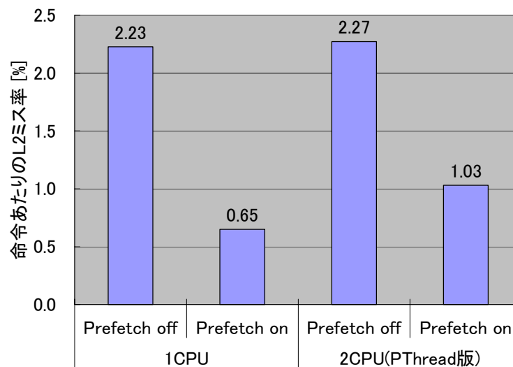
図 1 姫野ベンチマークによるメモリプリフェッチの効果
