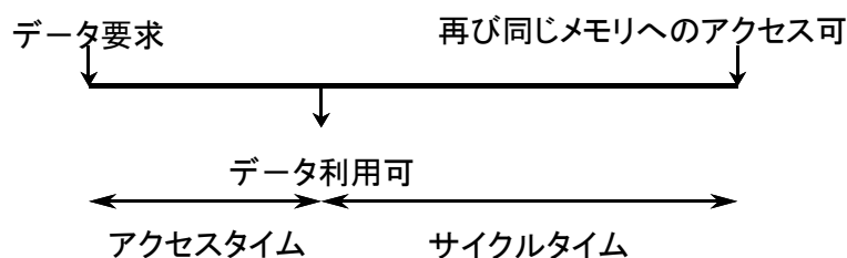
DRAMの動作
