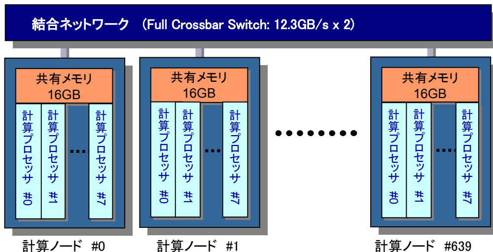
図 1 地球シミュレータのハードウェア構成
