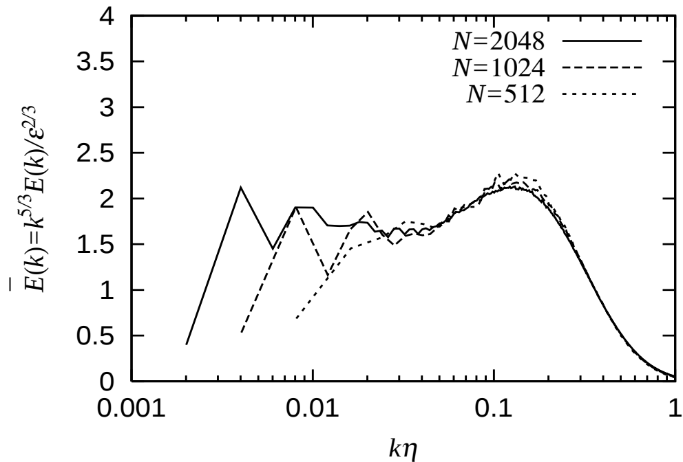
図 2 規格化した乱流場のエネルギースペクトル
