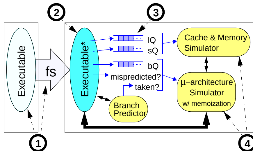
図 3 FastSim の構成[5]
